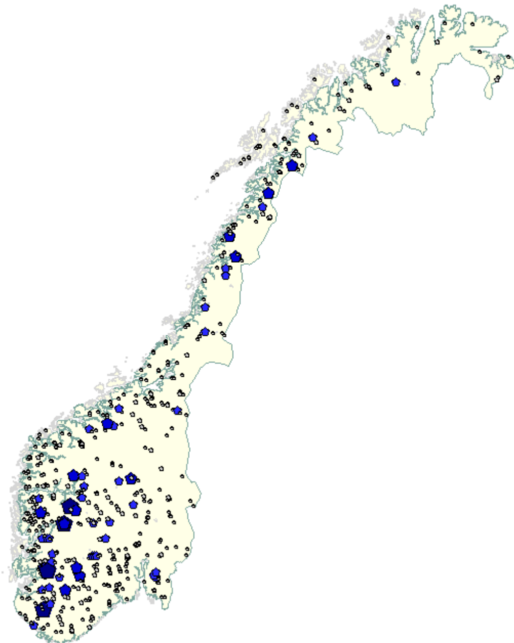
Figur 3.1 Produksjonsanlegg i det norske kraftsystemet. De tre ulike mørkeblå symbolene angir anlegg med h.h.v. 500-1240, 250-500 og 120-250 MW installert ytelse, etter avtagende størrelse. (Kilde: Norsk Kraftforsyning FFI/Rapport-2000/04450)
